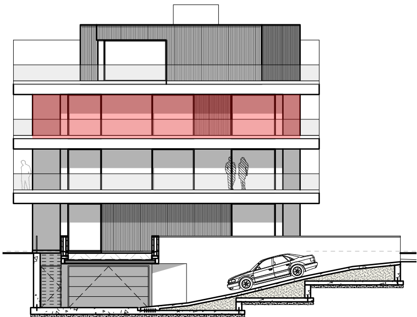
ZIJGEVEL LINKS
