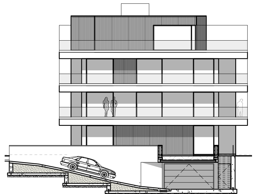
ZIJGEVEL RECHTS
