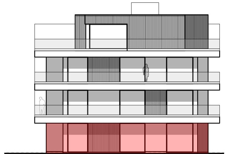
ZIJGEVEL LINKS
