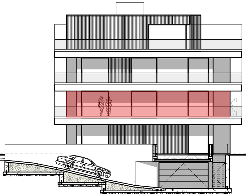
ZIJGEVEL RECHTS
