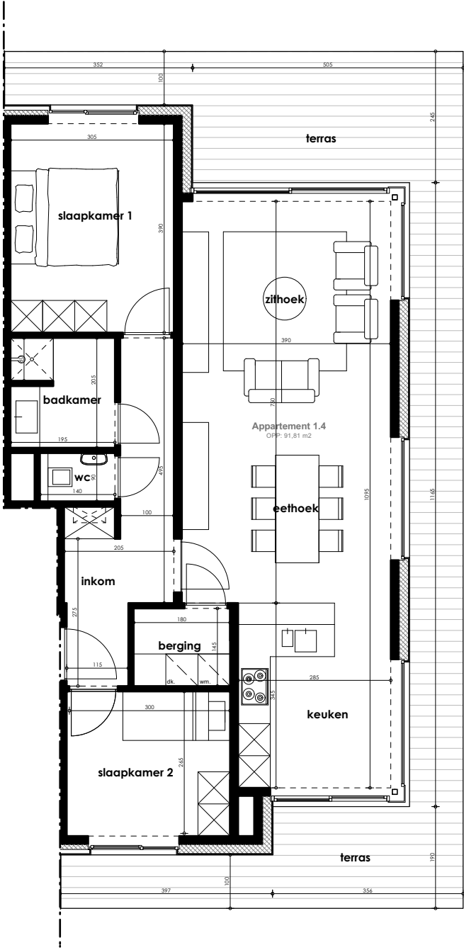
GRONDPLAN
