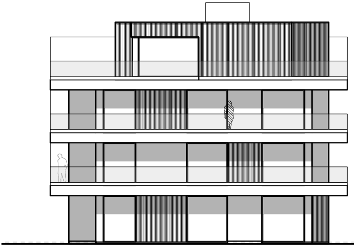
ZIJGEVEL LINKS
